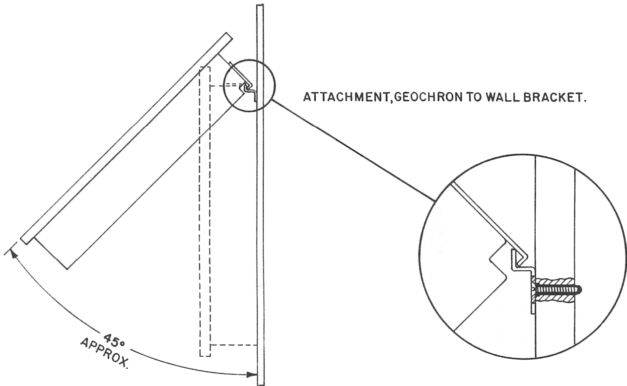
図4 本体を金具に引っ掛ける
