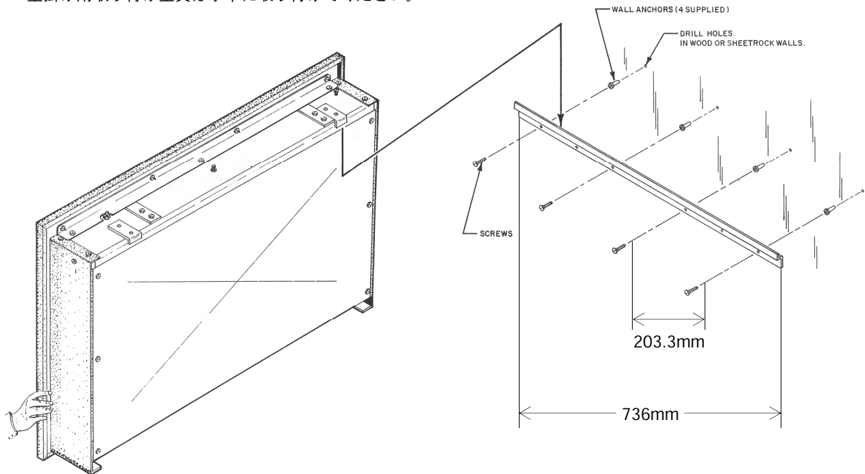
図3 取り付け図
