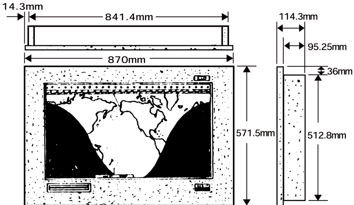
図5 外形寸法
