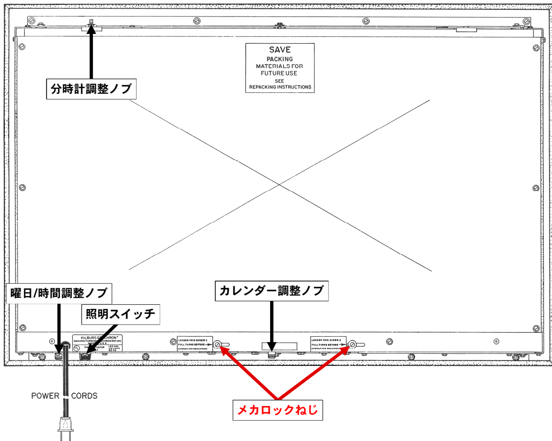
図1 本体背面図
